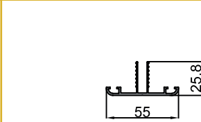
10-10099 Taşıyıcı Profil Orta Kapağı Carrier Profile Middle Cover 0,472 kg/m
