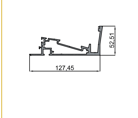
10-10451 Cam Taşıyıcı Profil / Glazing Carrier Profile 2.362 kg/m
