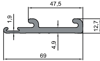
35-5355 Kiremit Çatı Kancası Profili/ Tile Roof Hook Profile 1.078 kg/m
