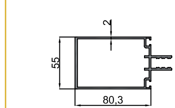
10-10097 Polikarbon Taşıyıcı Profil /Polycarbonate Carrier Profile 1.851 kg/m
