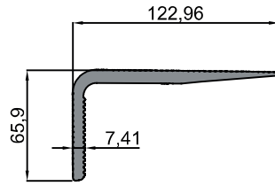
35-5355 Kiremit Çatı Kancası Profili/ Tile Roof Hook Profile 1.078 kg/m
