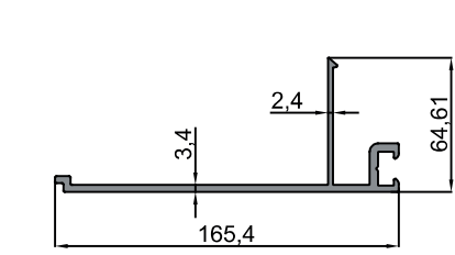
10-10098 Cam Taşıyıcı Profil/Glazing Carrier Profile 2.194 kg/m
