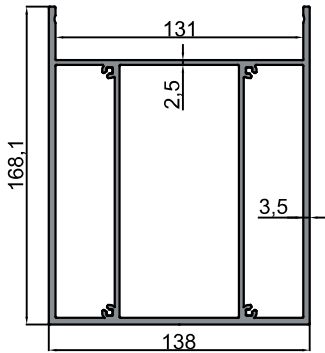
10-10060 Duvar ve Oluk Profili Kapağı Wall and Gutter Profile Cover 0.744 kg/m
