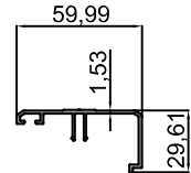
10-10556 Taşıyıcı Profil Yan Kapağı Carrier Profile Side Cover 0.531 kg/m
