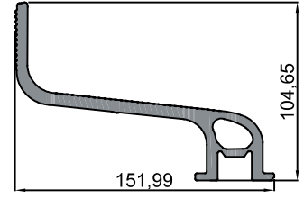
35-5366 Kiremit Çatı Alt Kasa Profili / Tile Roof Bottom Frame Profile 5.041 kg/m
