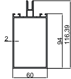
10-10556 Taşıyıcı Profil Yan Kapağı Carrier Profile Side Cover 0.531 kg/m
