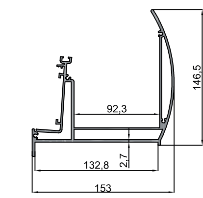
10-10285 Duvar ve Oluk Profili İç Kapağı /Wall and Gutter Profile Inside Cover 0.577 kg/m
