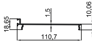
10-10534 Cam Taşıyıcı Profil E Glazing Carrier Profile E 2.691 kg/m
