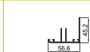
10-10100 Taşıyıcı Profil Yan Kapağı Carrier Profile Side Cover 0.659 kg/m
