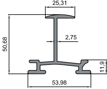
35-5364 Kiremit Çatı İç Bağlantı Profili/ Tile Roof Internal Connection Profile 0.625 kg/m
