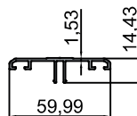
10-10551 Taşıyıcı Profil Orta Kapağı Carrier Profile Middle Cover 0.450 kg/m
