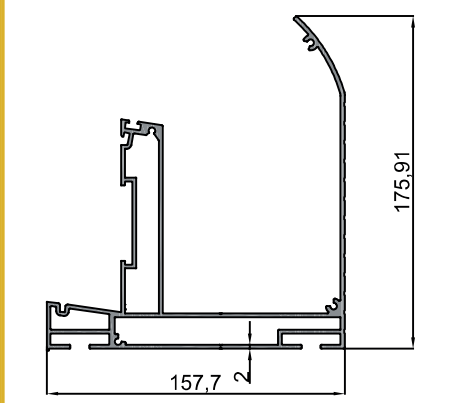
10-10455 Oluk ve Duvar Profili Kapağı Gutter and Wall Cover Profile 0.544 kg/m
