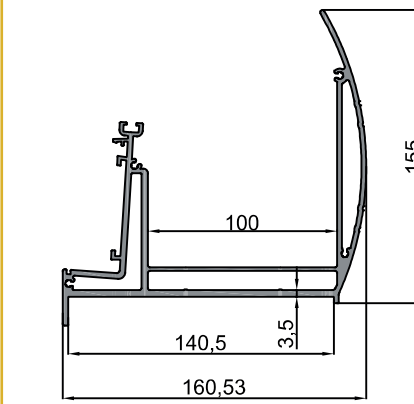
10-10284 Oluk Profili Dış Kapağı /Gutter Profile Outside Cover 1.402 kg/m
