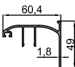
10-10061 Taşıyıcı Profil Yan Kapağı Carrier Profile Side Cover 0.754 kg/m
