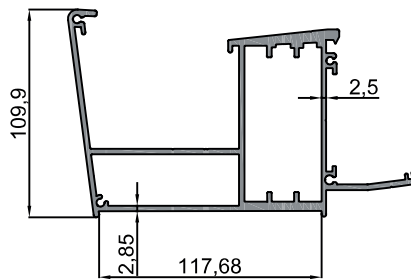
10-10057 Oluk Profili / Gutter Profile 5.704 kg/m
