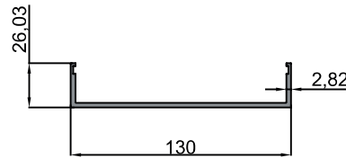
10-10057 Oluk Profili / Gutter Profile 5.704 kg/m
